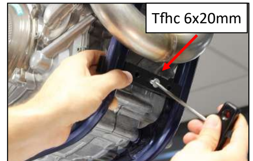
The 8mm plate has to be placed with the chamfered sides going inside of the frame and will be fixed by auto drilling in the 20mm part. La plaquette 8mm doit être placée avec les côtés chanfreinés à l'intérieur du cadre et fixée par auto perçage dans la bride 20mm
