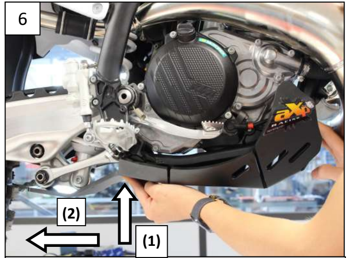
(1) Push to the top , (2) push to the rear (1) Pousser vers le haut, (2) Pousser vers l'arrière
