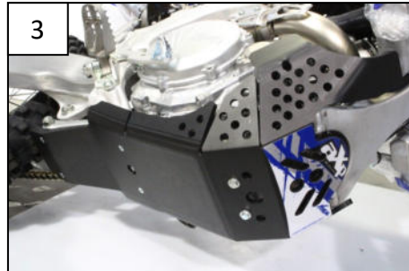
Fix the rear & then the front Fixer l'arrière puis l'avant
