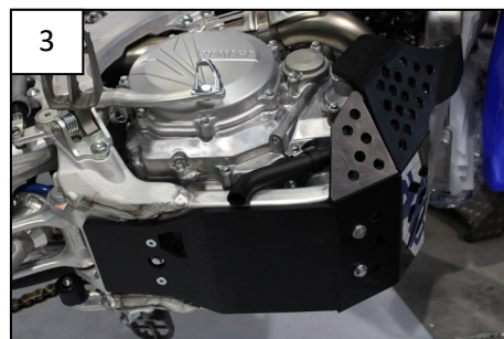
Fix the rear&front of the skid plate Fixer l'avant & l'arrière du sabot
