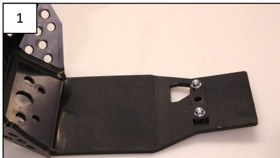
Fit the rear plastic part Fixer la pièce plastique arrière
